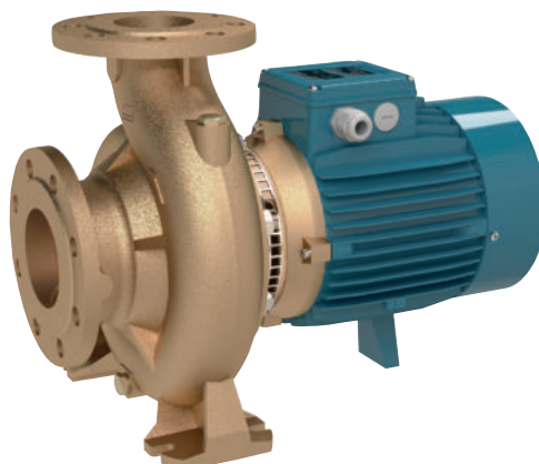
BNM, BNM4 (Ausführung Blockbauweise in Bronze)
