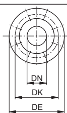
Flansche nach EN 1092-2
