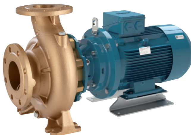
NMS, NMS4 (Ausführung Steckwellenkonstruktion in Grauguss) BNMS, BNMS4 (Ausführung Steckwellenkonstruktion in Bronze)
