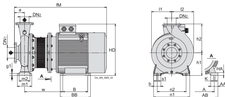
Flansche nach EN 1092-2
